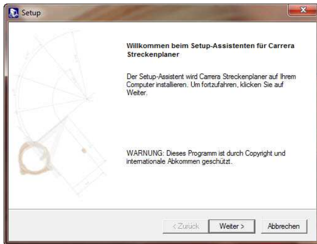
Abbildung 1: Installationsassistent
